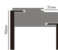
Type 4 Κάσωμα ίσιο, φαρδύ περβάζι, πρόσωπο / Straight frame form with wide architrave outside
