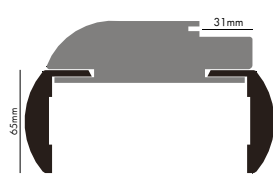
Type 2 Κάσωμα οβάλ Rounded frame form
